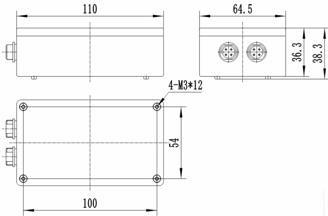
数据采集单元外观尺寸图
