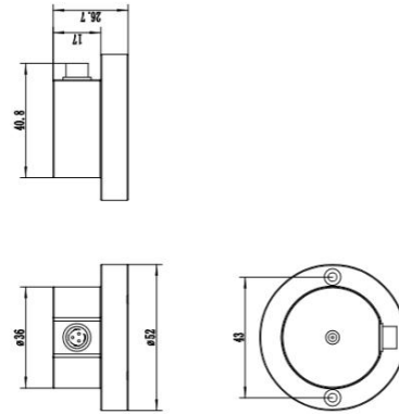
声音传感器外观尺寸图
