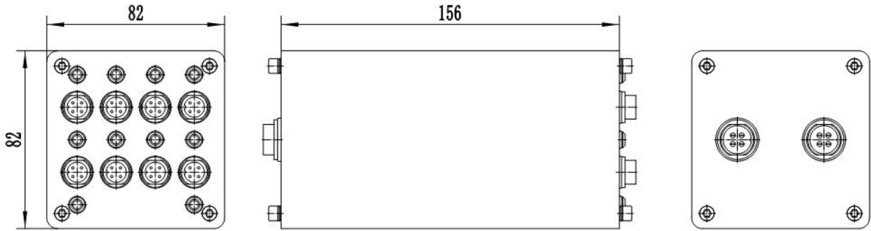
KZC12 硬件尺寸图
