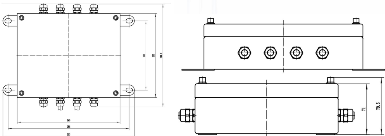
ZJS12-Z 硬件尺寸图
