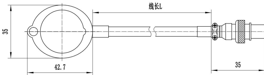
KZC12 硬件尺寸图
