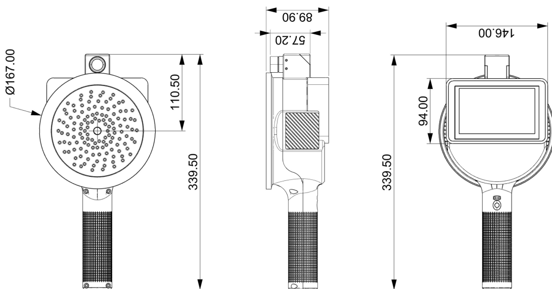
XS-SN-7FB11 产品外观图
