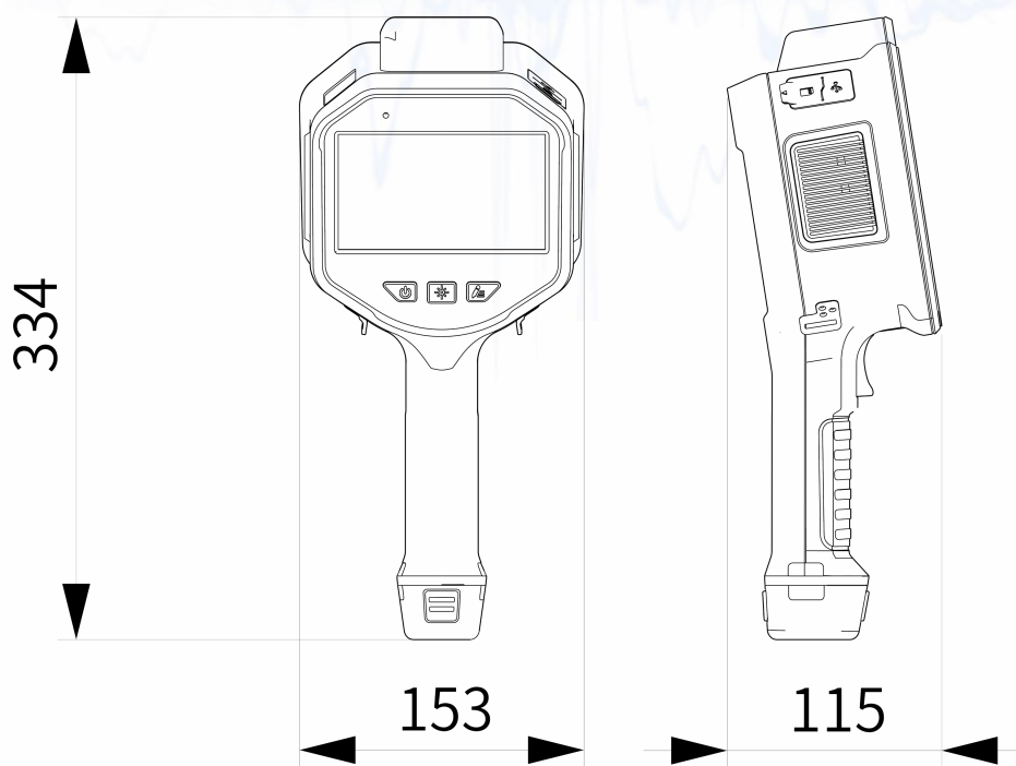
XS-SC60 产品外观
